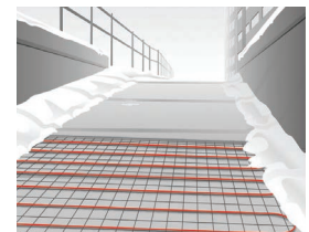
Freiflächenbeheizung für Rampen usw.
